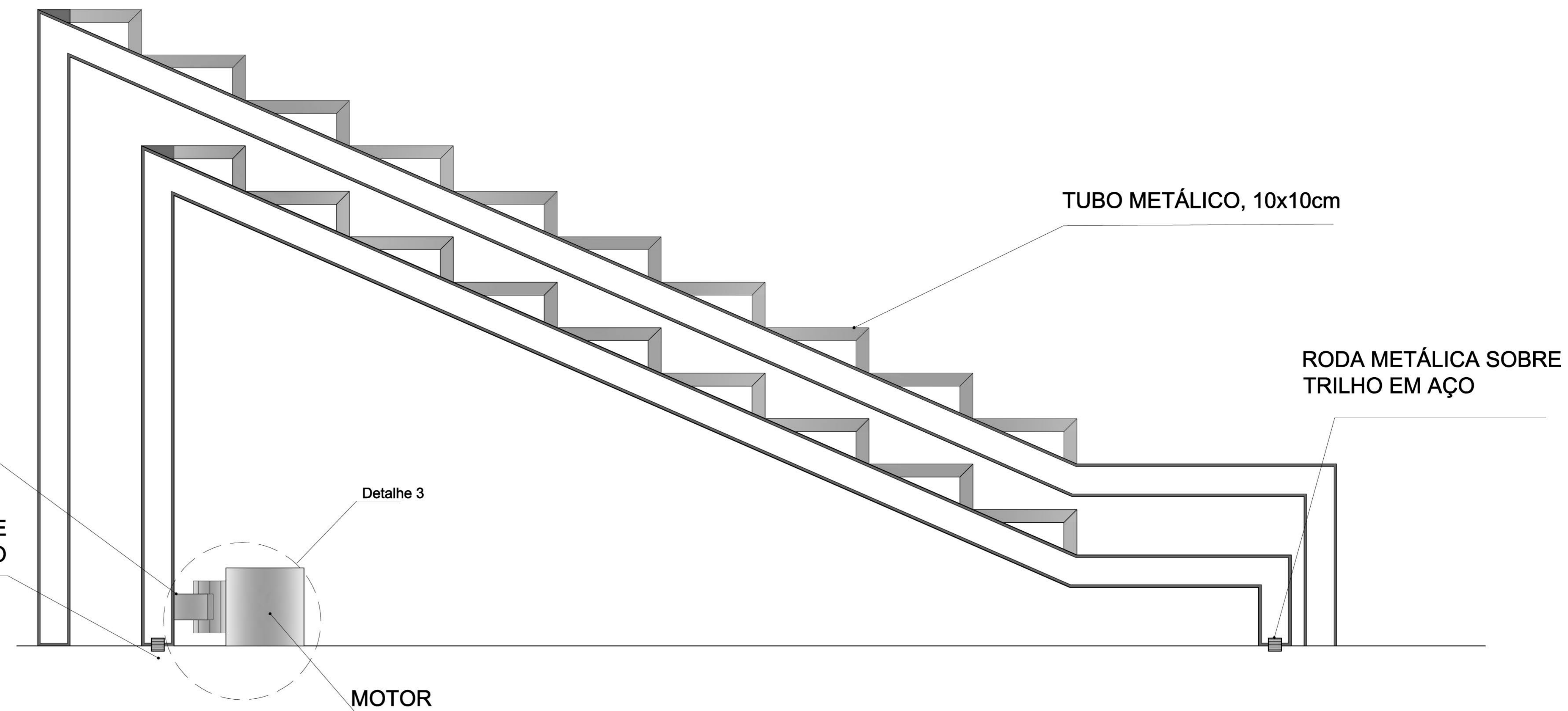
DETALHE DAS ARQUIBANCADAS Detalhe 4 esc. 1:20
