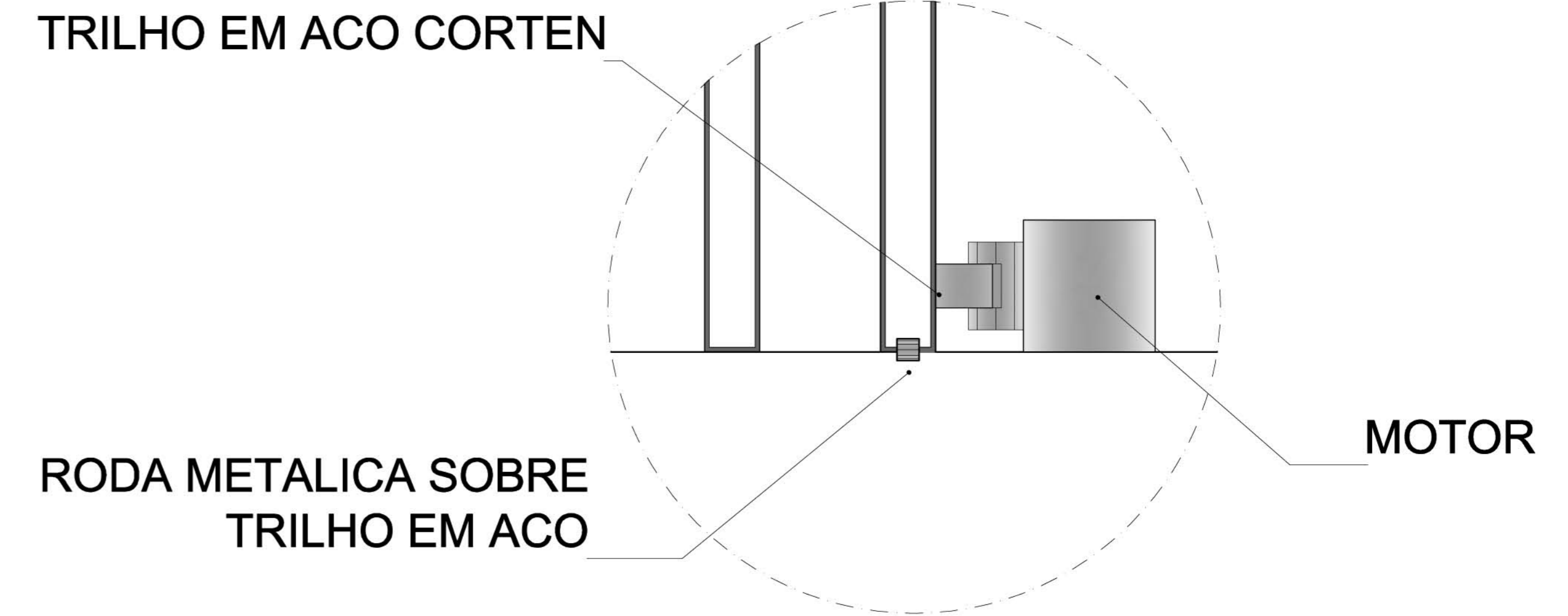
DETALHE DAS ARQUIBANCADAS Detalhe 4 esc. 1:20
