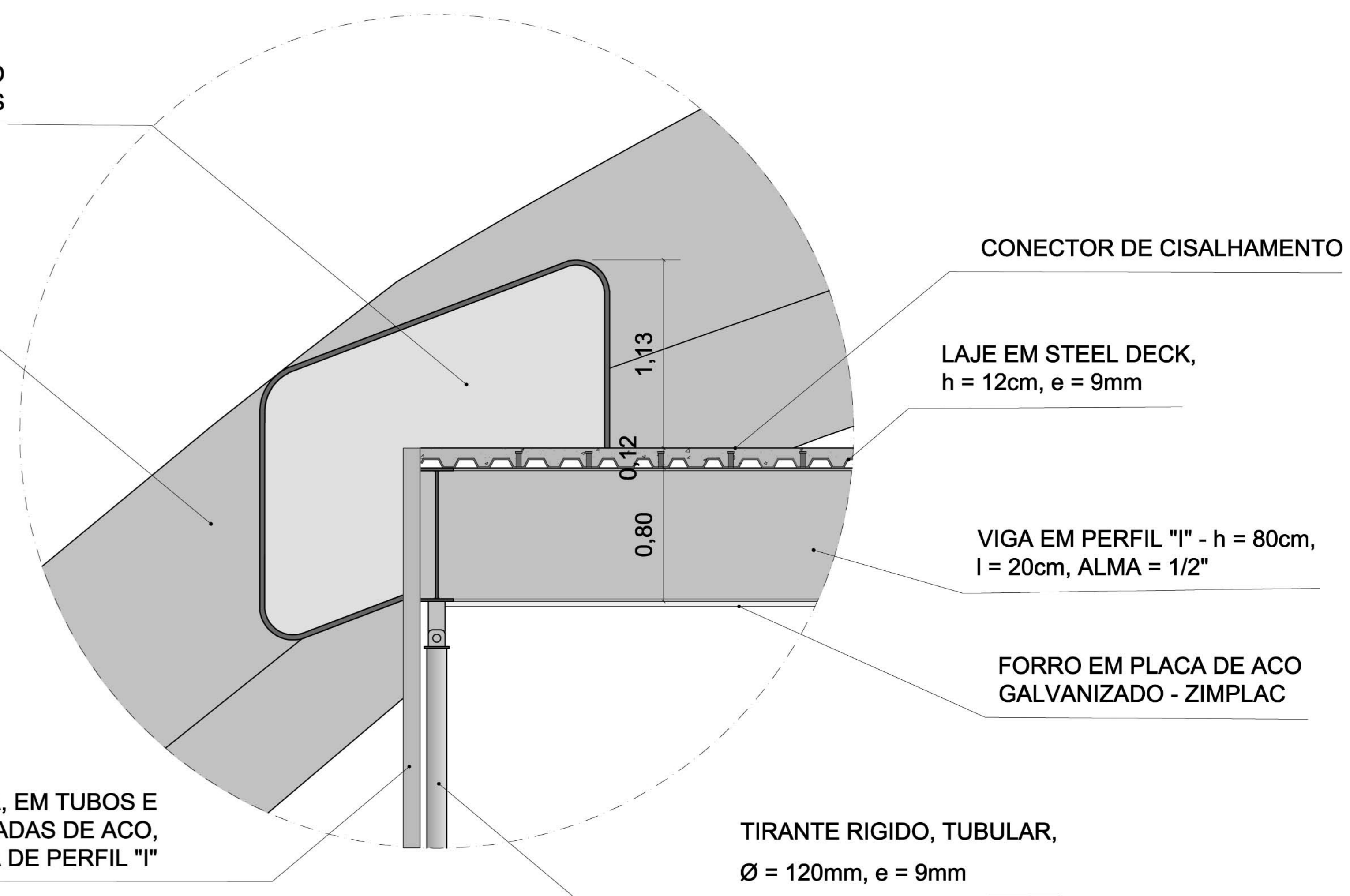
ENGASTE VIGA - PERFIL METÁLICO Detalhe 3 esc. 1:20
