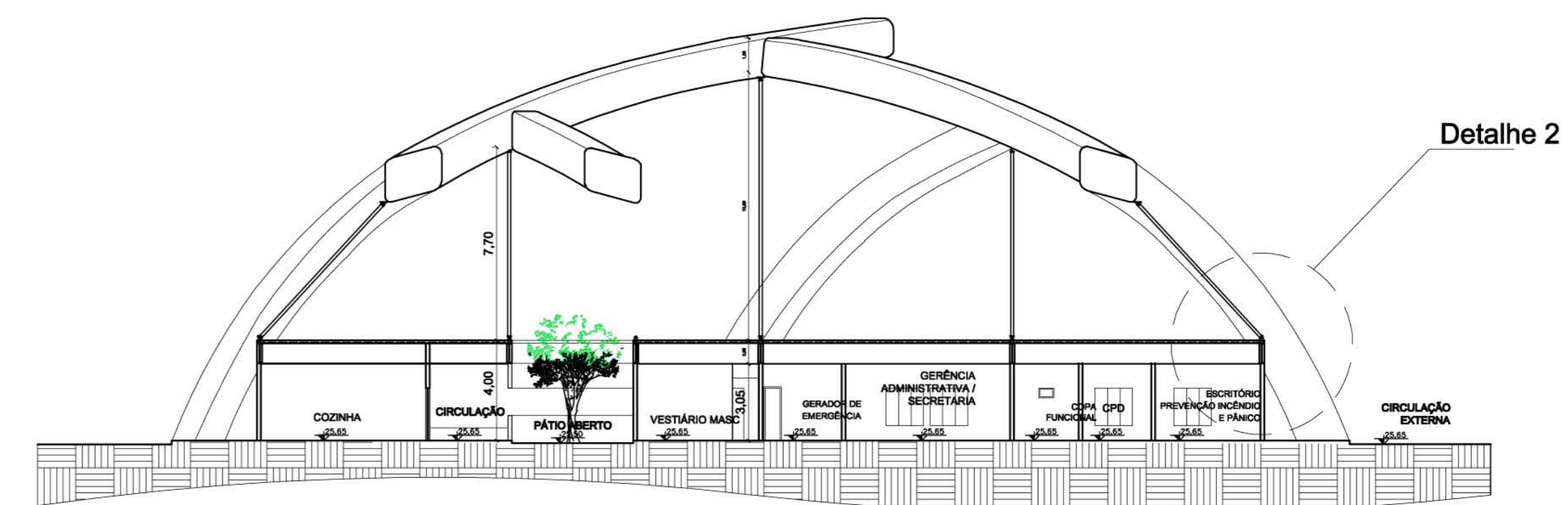
ADMINISTRAÇÃO Corte esc. 1:200 AA
